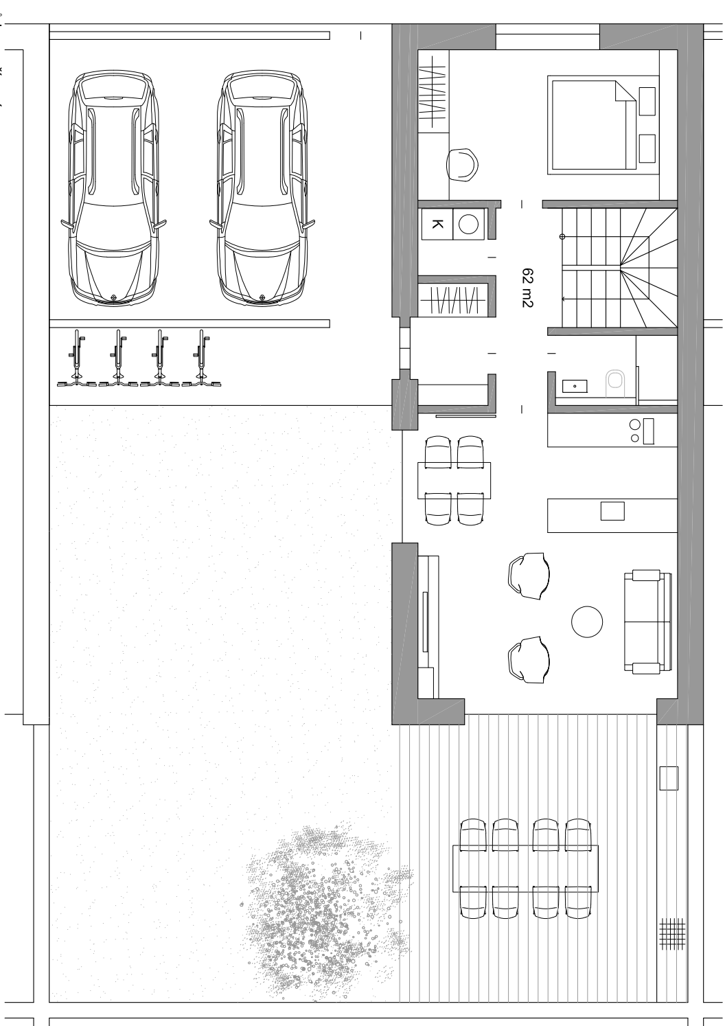
půdorys přízemí
