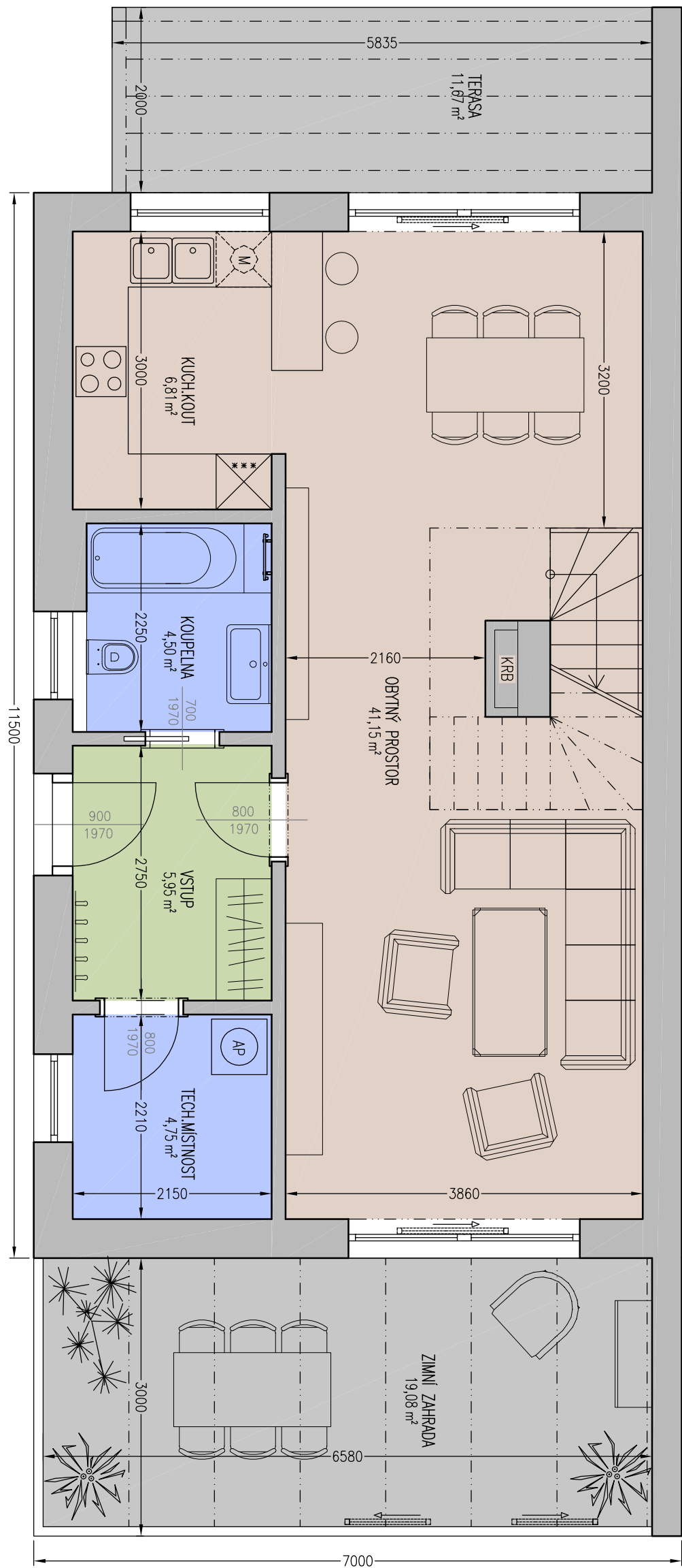
Půdorys 1.NP
