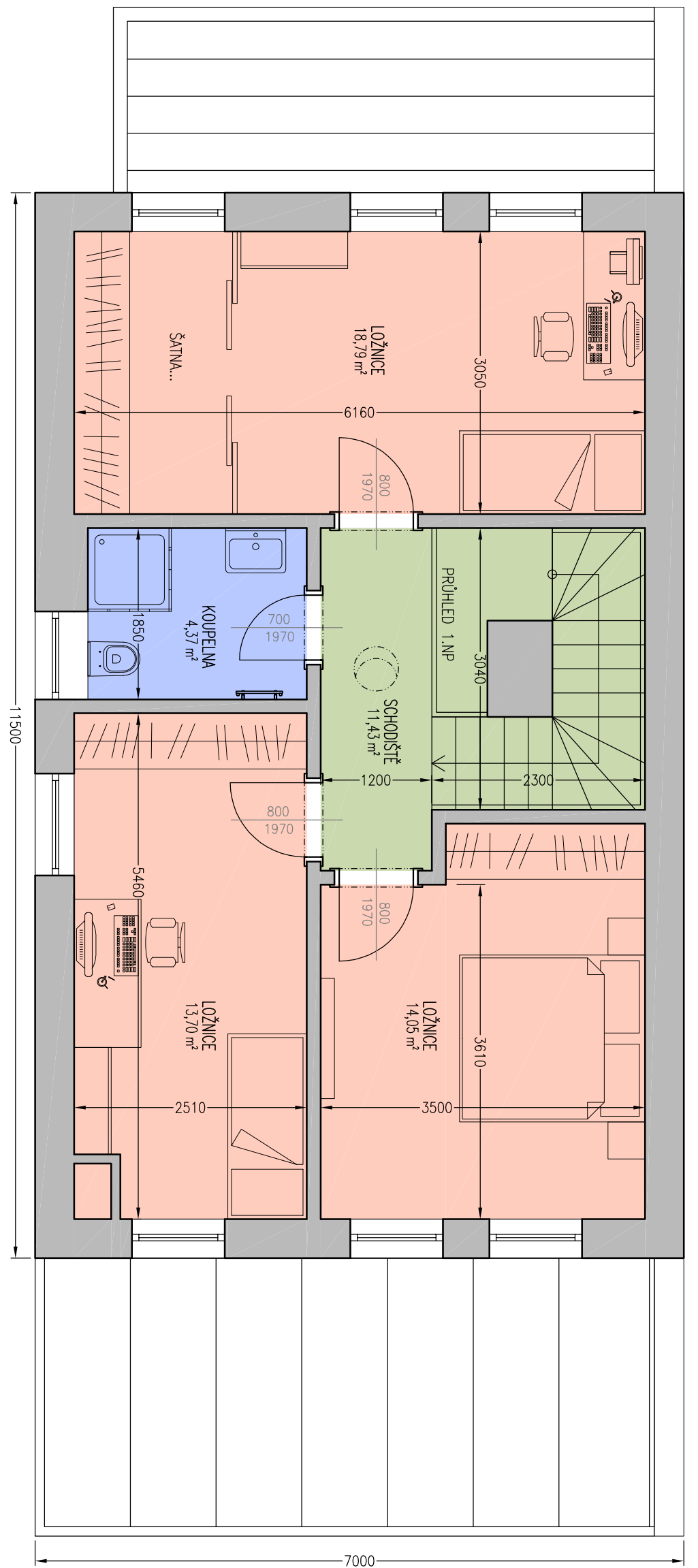
Půdorys 2.NP
