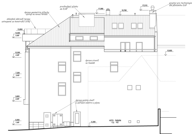
POHLED VÝCHODNÍ - NAVRHOVANÉ ÚPRAVY
