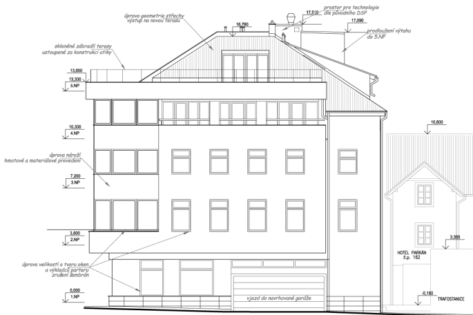
POHLED JIŽNÍ - NAVRHOVANÉ ÚPRAVY
