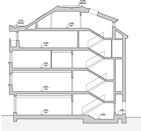
TYPICKÝ ŘEZ OBJEKTEM - STAV DLE VYDANÉHO STAVEBNÍHO POVOLENÍ
