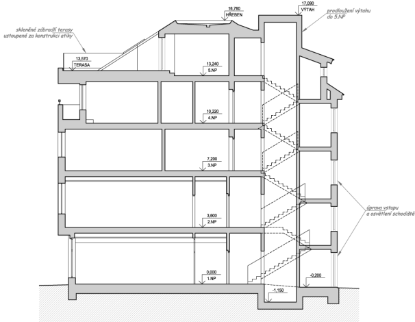
TYPICKÝ ŘEZ OBJEKTEM - NAVRHOVANÉ ÚPRAVY
